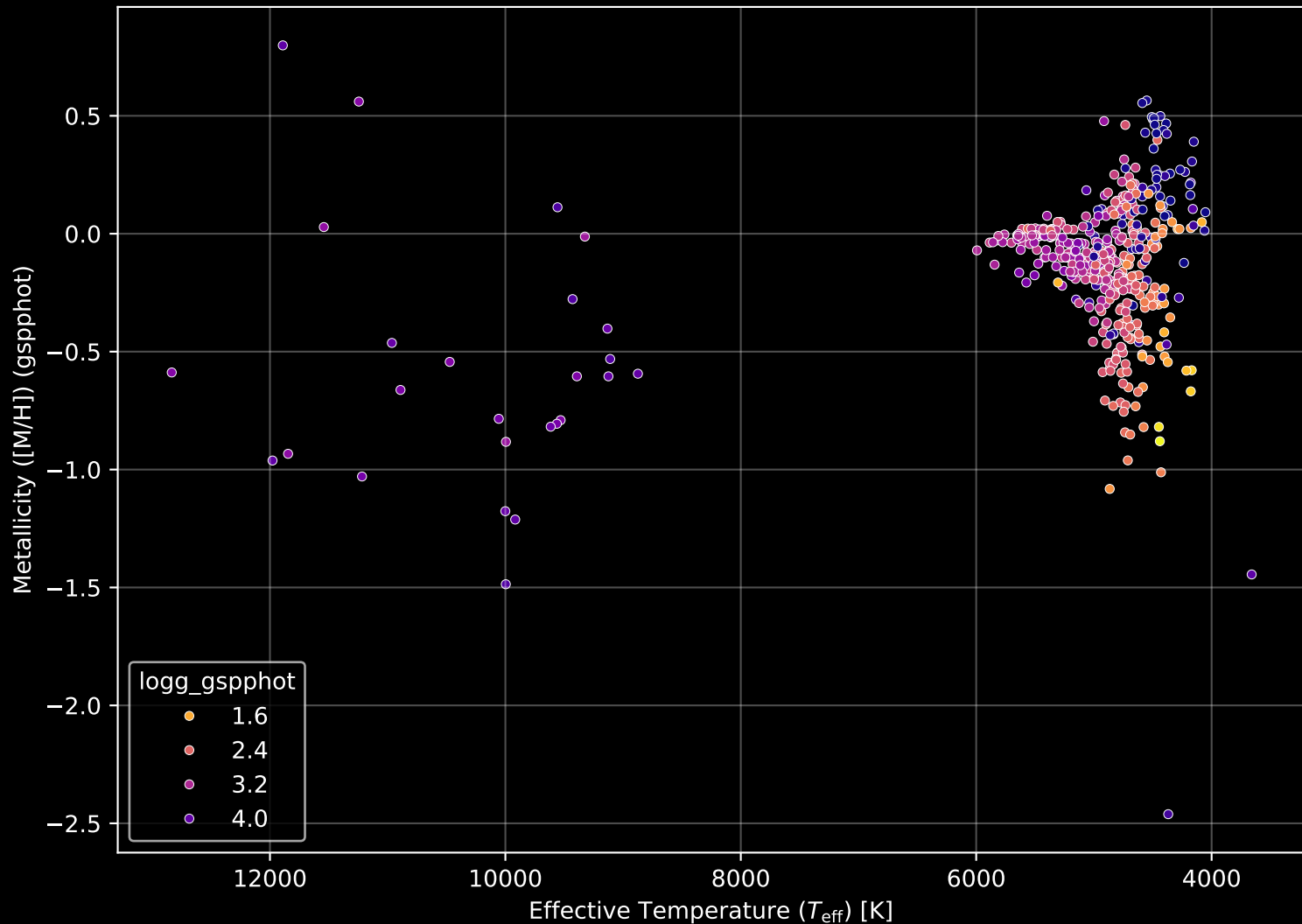
APOGEE DR17 Field: [210+08] Stellar Population Parameters (n= 512)
